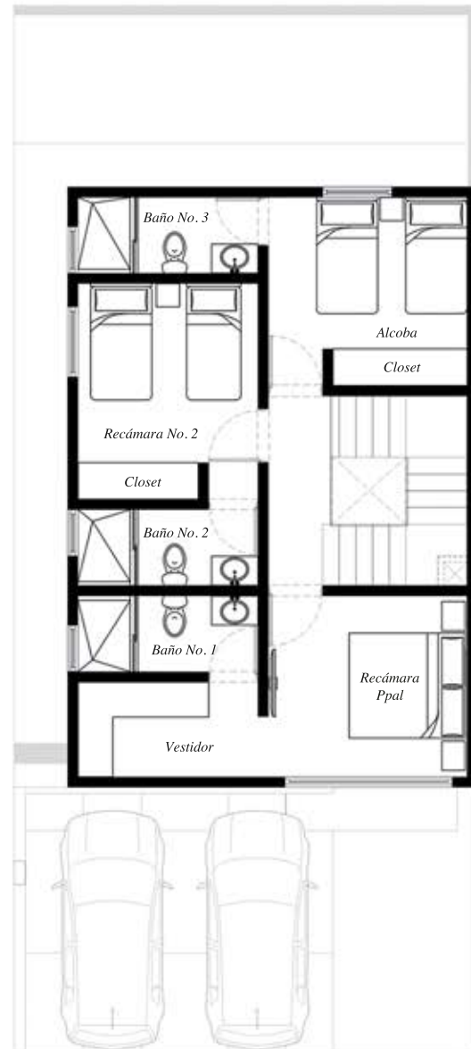
PLANTA ALTA
